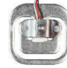
Resim 5.20: Ağırlık algılayıcı
