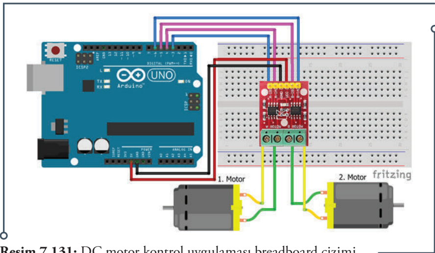
Resim 7.131: DC motor kontrol uygulaması breadboard çizimi
