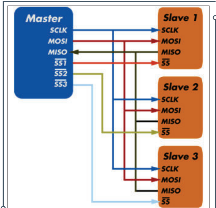
Resim 7.116: SPI veri yolu bağlantı şekilleri
