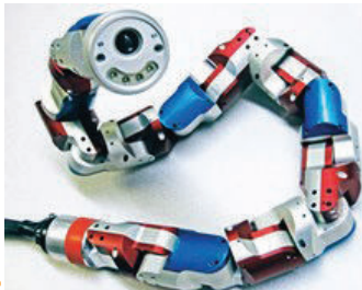
Resim 2.16: Yılan robotlar
