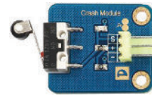
Resim 5.25: Çarpma algılayıcı
