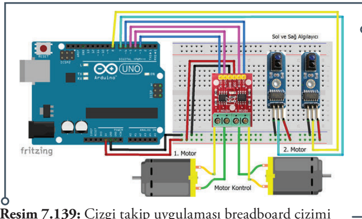
Resim 7.139: Çizgi takip uygulaması breadboard çizimi
