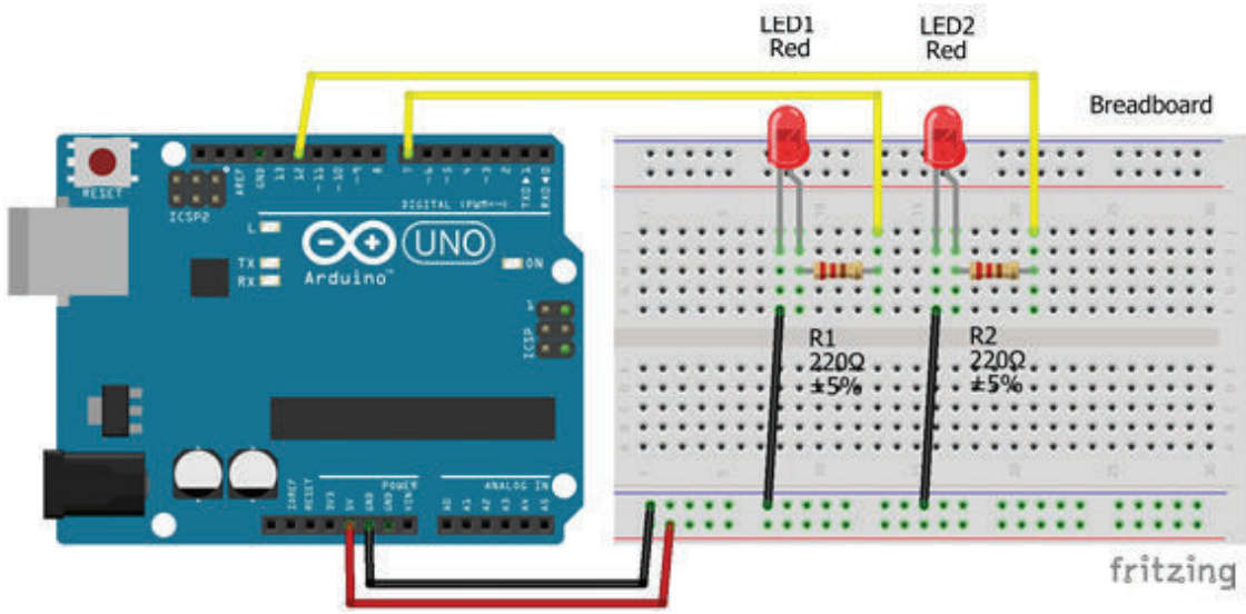
Resim 6.44: Arduino UNO ile LED uygulaması Breadboard çizimi
