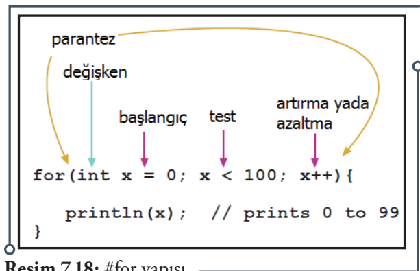
Resim 7.18: #for yapısı
