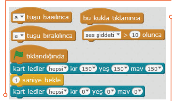
Resim 6.30: Olay örneği
