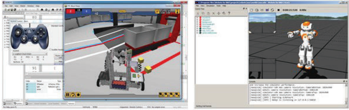
Resim 2.9: Sanal robotlar
