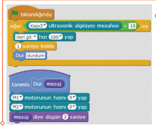
Resim 6.28: Parametre örneği
