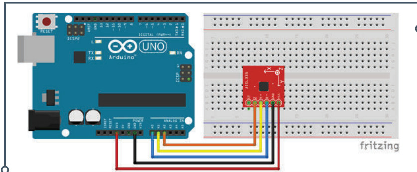
Resim 7.137: İvmeölçer uygulaması breadboard çizimi
